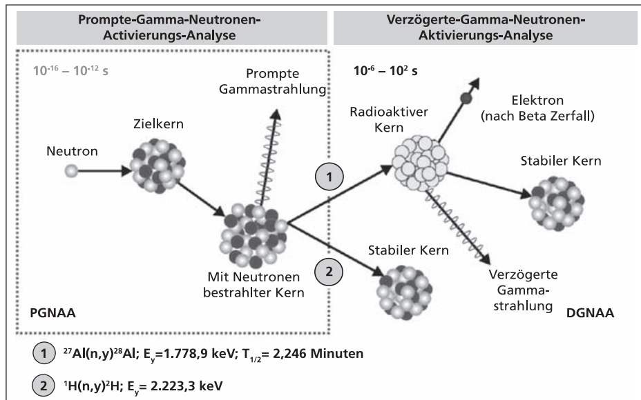
Abbildung 2: Prinzip der Prompten-Gamma-Neutronenaktivierungsanalyse
