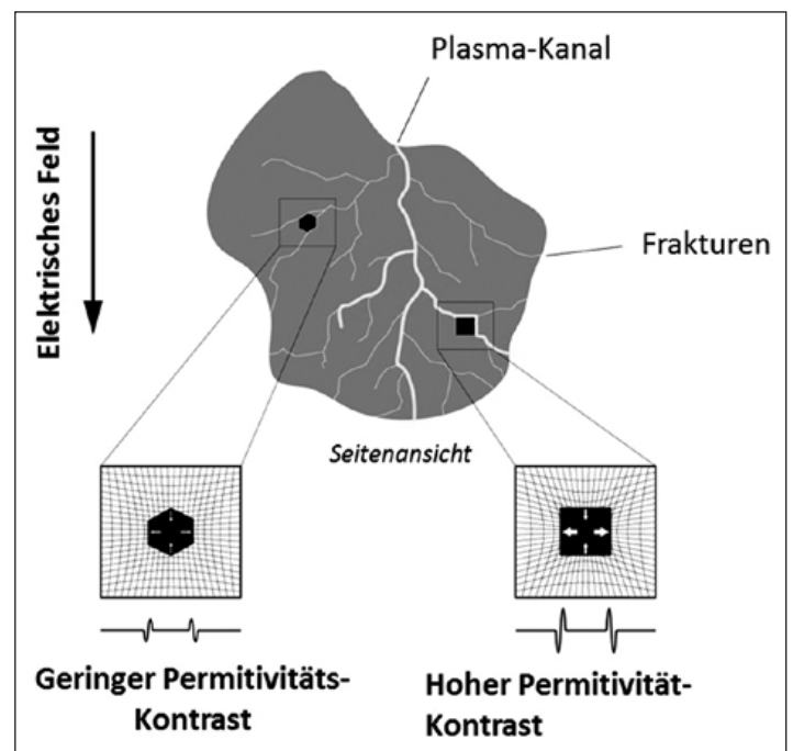
Abbildung 6: Ausbildung eines Plasmakanals Quelle: Selfrac AG
